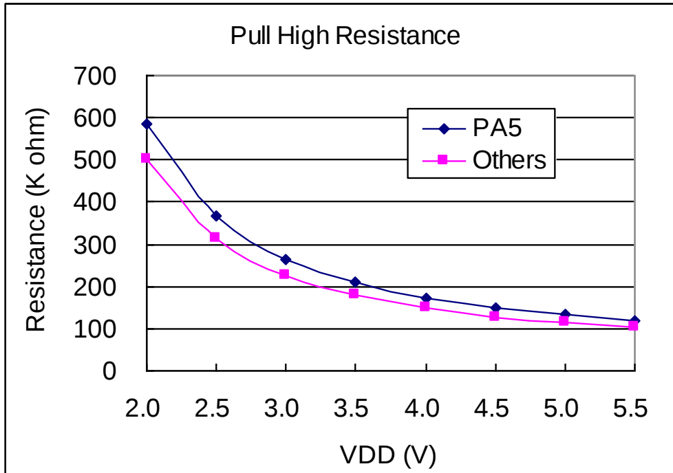
4.14. IO 引脚上拉阻抗曲线图
