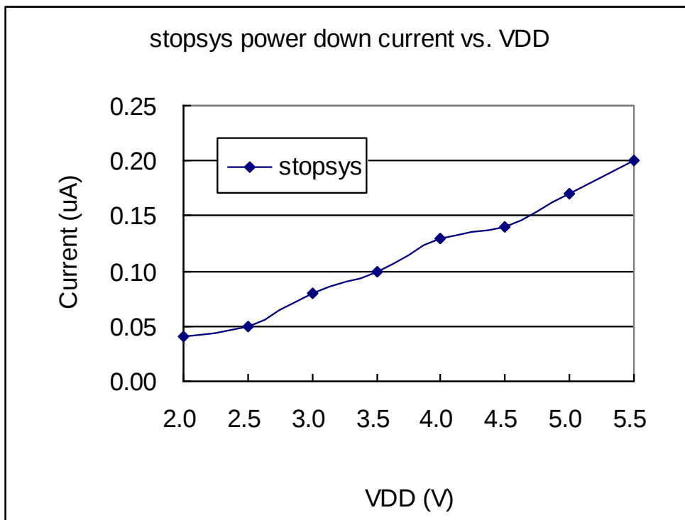
4.15. 掉电电流( I_{PD} ) / 省电电流 ( I_{PS} ).vs VDD 关系曲线图
