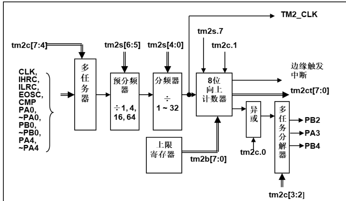
图 10: Timer2 硬件框图
