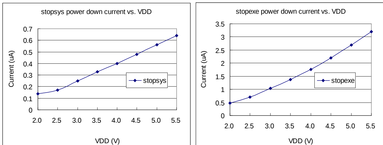
4.15. 掉电消耗电流( I_{PD} )与省电消耗电流( I_{PS} )关系曲线图
