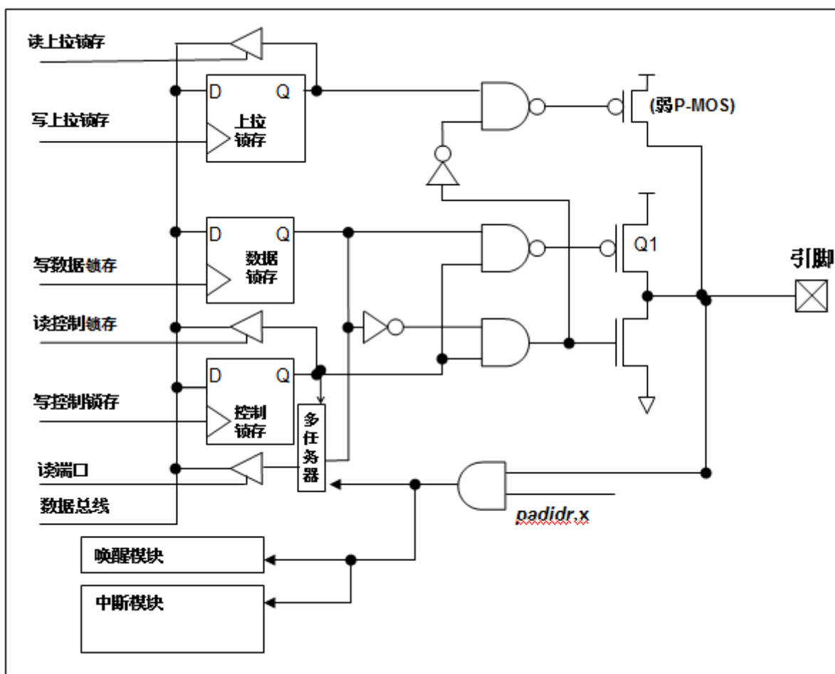
图 13: 引脚缓冲区硬件图
