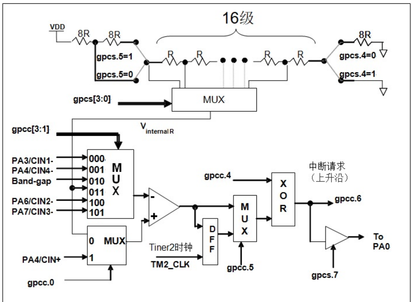
图 3: 比较器硬件图框
