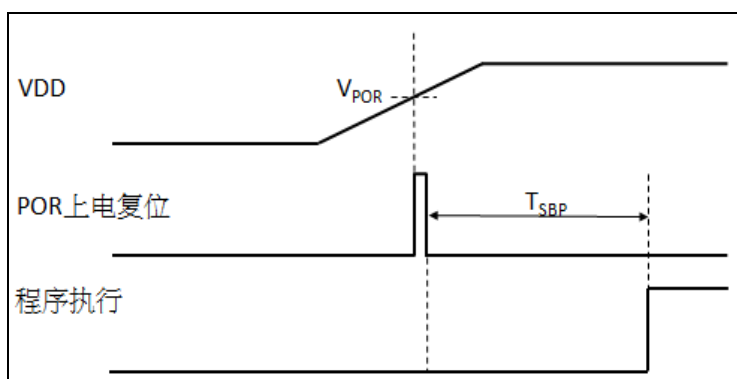
图 1: 上电复位时序
